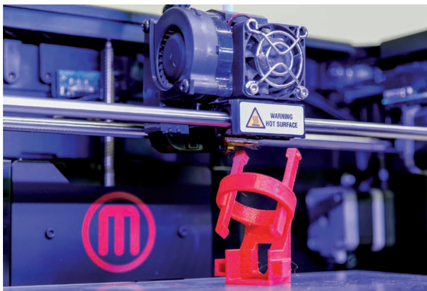
Mit einem 3D-Drucker wurde der Halter für eine Datenbrille erstellt.
