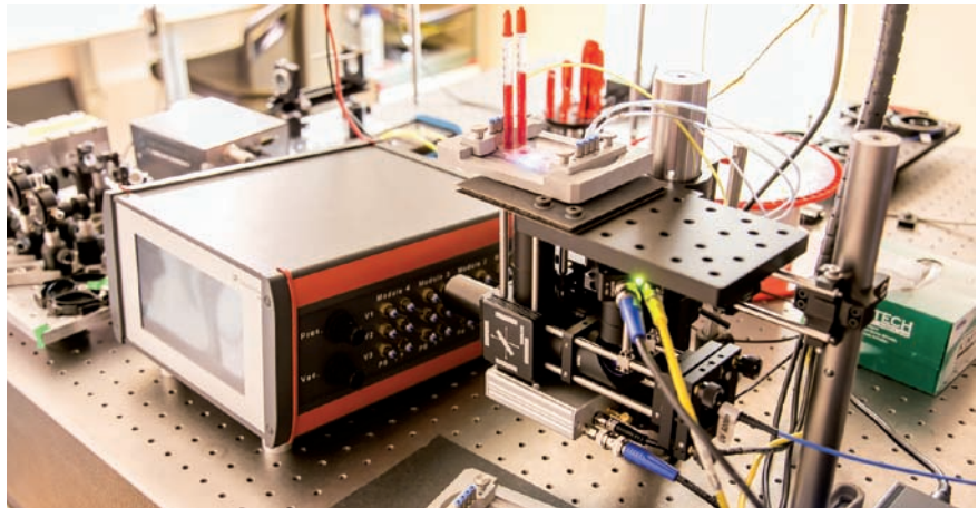
Links im Bild ist die Pumpensteuerung des Bioreaktors zu sehen, die für die gezielte Nährstoff- und Testsubstanzen-Durchströmung zuständig ist. Rechts ist der Laboraufbau des optischen Messsystems zur Erkennung des Lebenszustands der Zellen zu sehen.
