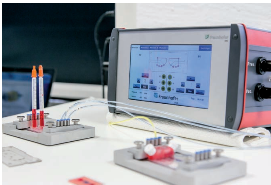
Das Bild zeigt ein automatisiertes Steuermodul zur Medienaktuierung (rechts) und universelle, mikrophysiologische Lab-on-a-Chip-Plattform des Fraunhofer IWS mit adaptivem Zellkultursegment und integriertem künstlichen Gefäßnetzwerksystem (links und vorn).
