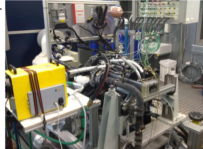
Motorenprüfstand
